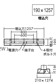
埋込型 DBL-31461 (100V) G ¥11,000 ランプ別梱包
