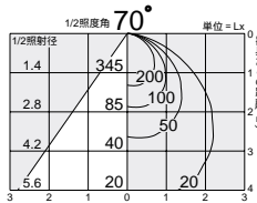
ミニクリプトン球100W 照明率表 P.950-F-
