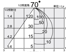
昼白色電球形蛍光灯(D形) 15W 照明率表 P.950-F-
