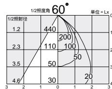
ミニクリプトン球60W 照明率表 P.951-A-
