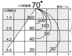
電球形電球形蛍光灯(D形) 25W 照明率表 P.950-F-
