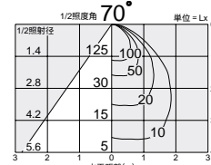
電球形電球形蛍光灯(D形) 15W 照明率表 P.950-F-
