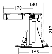
150 埋込穴
