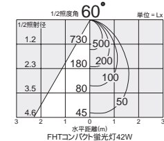
照明率表 P.946-B-4
