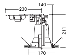
150 埋込穴
