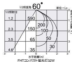
照明率表 P.946-C-3
