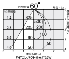
照明率表 P.946-C-2
