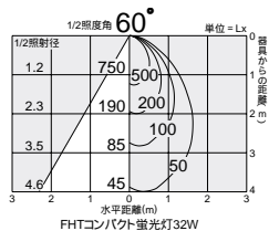
照明率表 P.946-C-1
