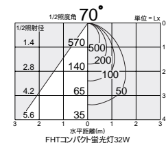
照明率表 P.946-C-4
