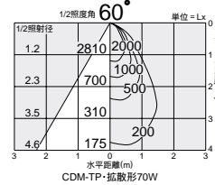
照明率表 P.944-D-1
