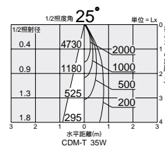
照明率表 P.944-F-
