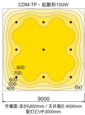
作業面照度分布図 DDL-51083
