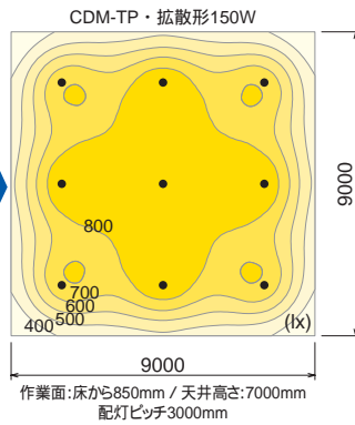
作業面照度分布図 DDH-3075XW
