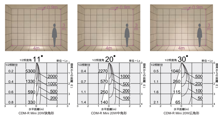
照明率表 P.942-C-1 照明率表 P.942-C-2 照明率表 P.942-C-3
