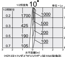
25ミ径12Vダイクロハロゲン球20W狭角形 照明率表 P.948-F-
