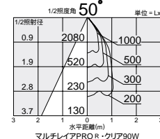
マルチレイアPRO R・クリア90W 照明率表 P.948-F-
