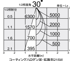
コーティングハロゲン球・拡散形215W 照明率表 P.948-F-
