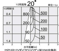
25ミ径12Vダイクロハロゲン球20W中角形 照明率表 P.948-F-
