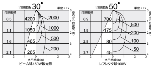
照明率表 P.950-B-
