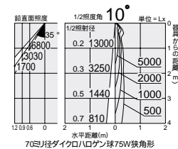
70ミ径ダイクロハロゲン球75W狭角形
