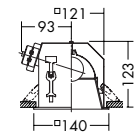
125 埋込穴
