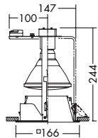
150 埋込穴
