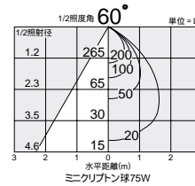
照明率表 P.949-E-1
