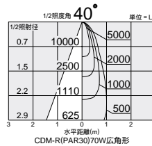
照明率表 P.949-D-1
