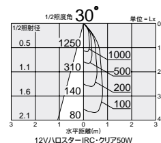
照明率表 P.942-A-4
