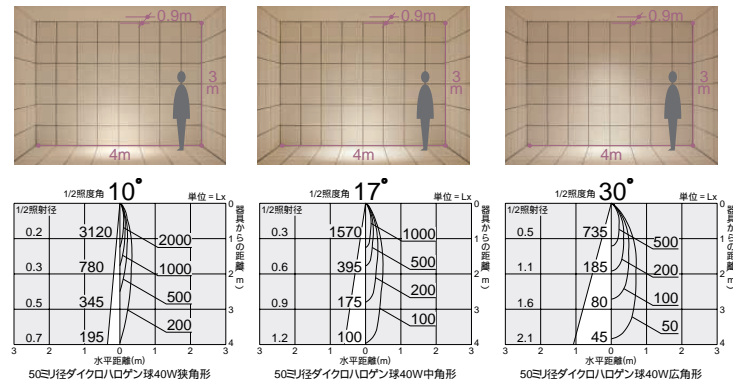
照明率表 P.949-F- 照明率表 P.949-F- 照明率表 P.949-F-
