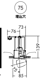
必要に応じて灯具が上下するため、壁面上部への照射が可能です。
