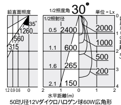
50ミ径12Vダイクロハロゲン球60W広角形
