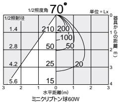
照明率表 P.949-E-1
