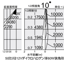
50ミ径12Vダイクロハロゲン球60W狭角形
