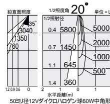
50ミ径12Vダイクロハロゲン球60W中角形
