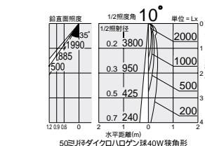
50mm径ダイクロハロゲン球40W狭角形
