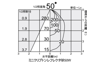
照明率表 P.951-B-1
