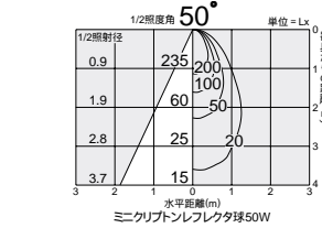
照明率表 P.951-B-1
