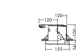
ダイクロハロゲン球 50W形 / 40W(径50mm) [3,000K]
