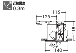
ミニクリプトンレフレクタ球 50W形 [2,800K]
