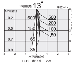
照明率表 P.950-D-
