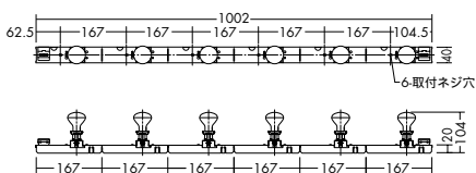
ミニクリプトン球 25W×6灯
