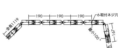
電球形蛍光灯(D形) 10W形
